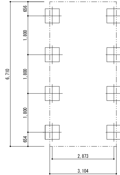
■ 基礎配置図
